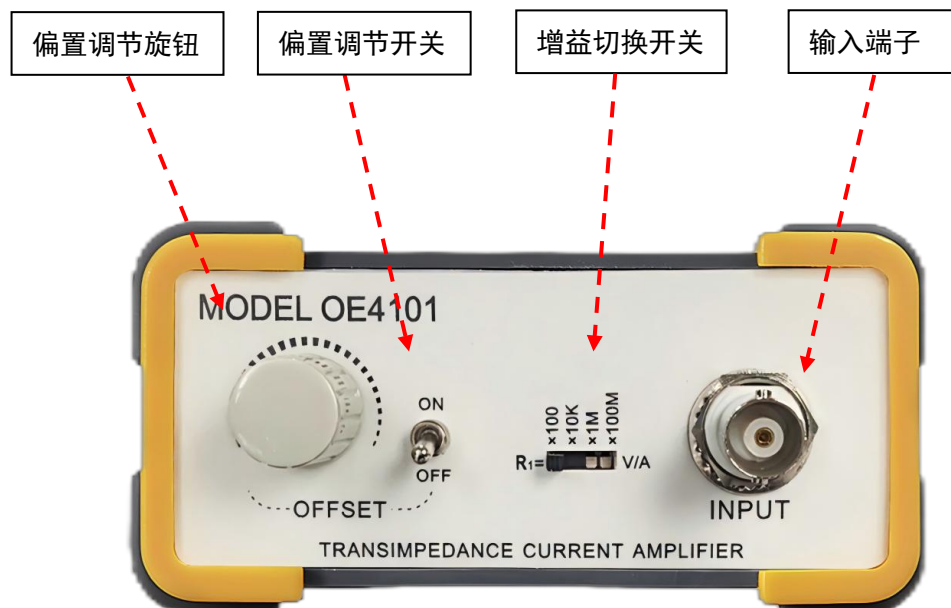
图 2. OE4101 主视图
