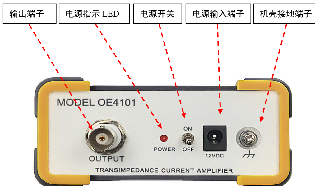
图 3. OE4101 背部视图
